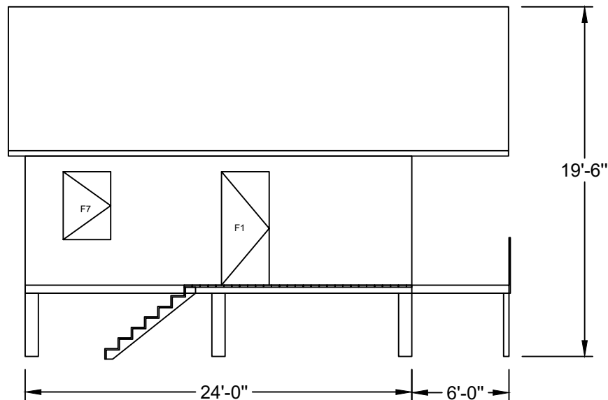
VUE LATÉRALE DROITE
