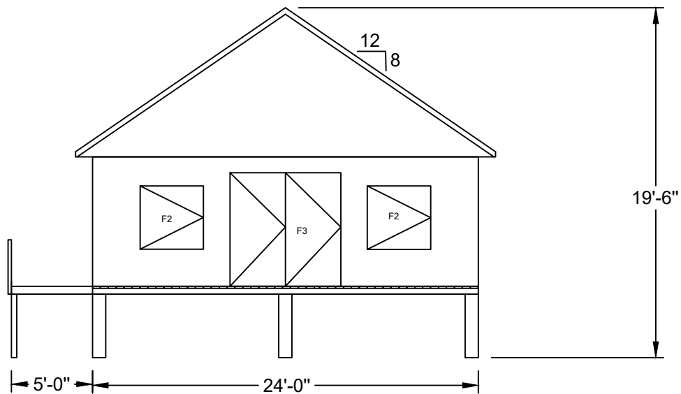
VUE AVANT
